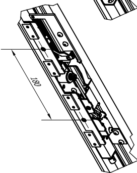
Version électrique menant avec option ré-armement Verrou 010 7 03 10 + Ré-armement 010 7 00 40
